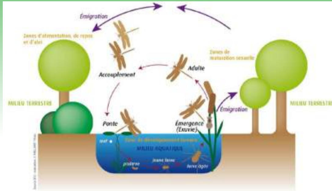
Schéma du cycle de vie des odonates. Source : Opie/SFO (2012).
